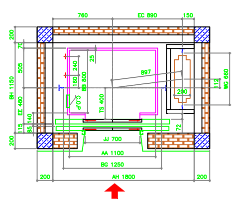
THANG TẢI KHÁCH ĐỐI TRỌNG ĐẶT BÊN HÔNG
